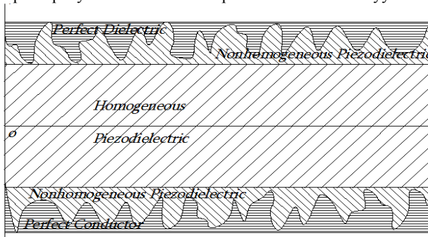
Рис. 3.1 Пятислойный композитный волновод с базовым однородным пьезоэлектрическим слоем с залитыми слабо неоднородными поверхностями
