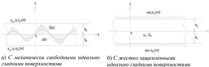
Рис. 2.1 Упругий слой-волновод из слабо неоднородного изотропного материала
