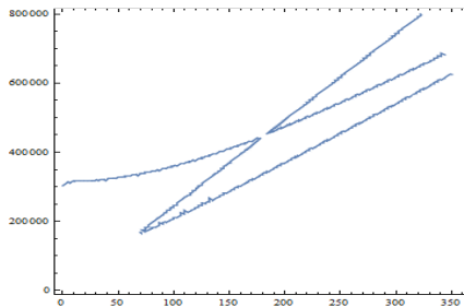
Рис. 3.3 б) Зависимость частоты \omega(k) быстрых коротких волн от волнового числа k \in [1.6; 350]
